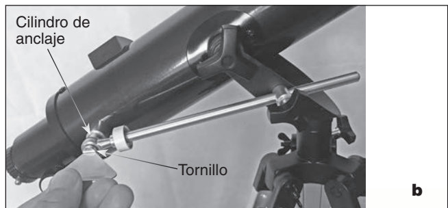
Figura 9. a) Inserte la barra de micromovimiento a través del agujero del receptáculo metálico de la montura de horquilla. b) Acople el otro extremo de la barra al cilindro de anclaje del tubo óptico.
