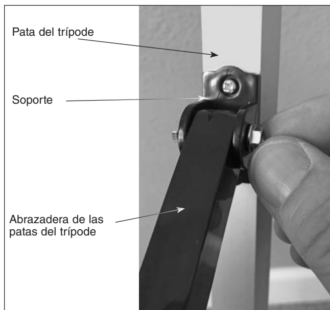
Figura 4. Fije la abrazadera de las patas del trípode al soporte en cada pata del trípode.
