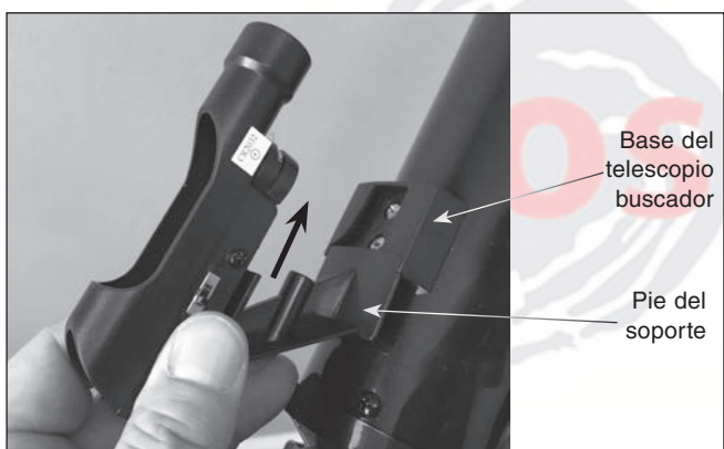
Figura 10. Inserte el soporte del telescopio buscador de punto rojo en la base cerca del enfocador como se indica.
