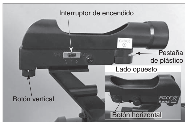
Figura 12. El telescopio buscador de punto rojo tiene botones de ajuste vertical y horizontal (insertado) para alinearlos con el telescopio.
