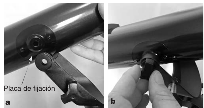
Figura 8. a) Coloque el tubo óptico en la montura de horquilla, alineando los agujeros de las placas de fijación del tubo con los de la montura de horquilla. b) Enrosque el botón de horquilla en el agujero roscado de las placas de fijación.
