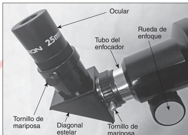
Figura 11. Sujete la diagonal estelar en el tubo del enfocador con el tornillo de mariposa del cuello del tubo y, a continuación, instale el ocular en la diagonal.
