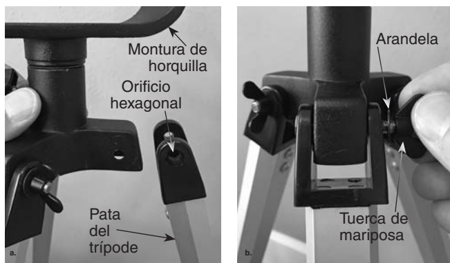
Figura 5. a) Acople las tres patas del trípode a la montura de horquilla, asegurándose de que la cabeza hexagonal del perno se apoya sobre el hueco hexagonal de la pata del trípode. b) Coloque una arandela y una tuerca de mariposa sobre el extremo expuesto del perno.
