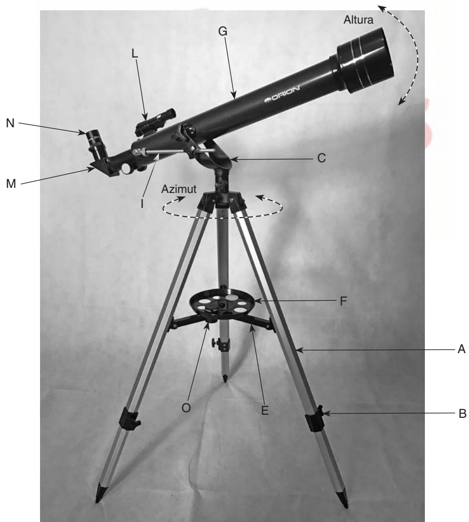
Figura 2. El telescopio altacimutal Observer II 60 mm completamente montado
