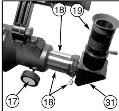
Fig. 1b: Enfocador, diagonal y ocular.
