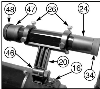
Fig. 1a: Ensamble del Enfocador
