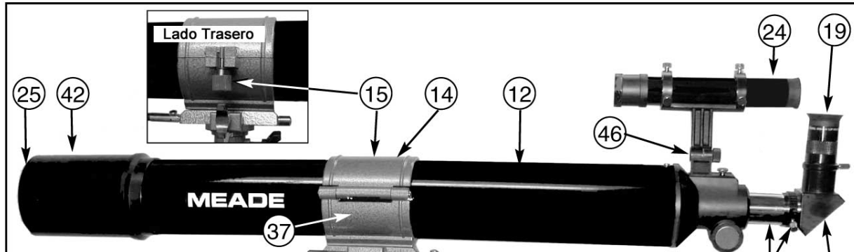
Fig. 1c: Montura ecuatorial
