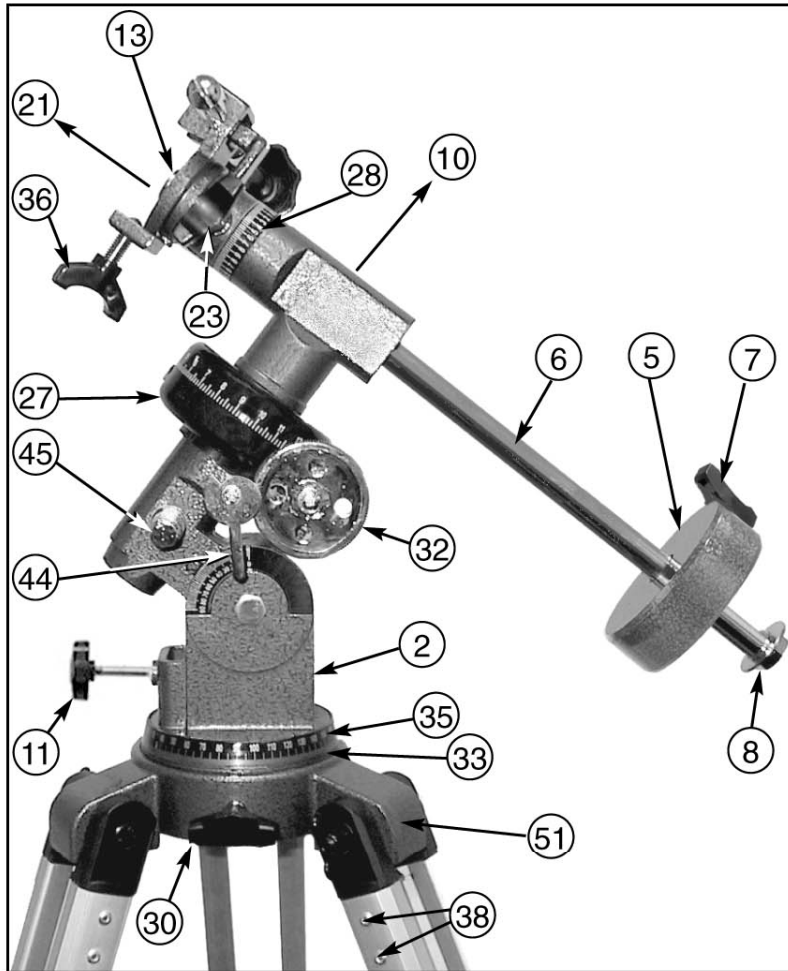
Fig. 1c: Montura ecuatorial
