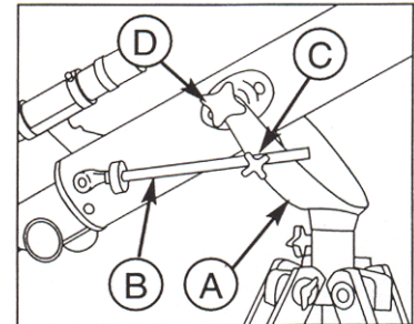
Fig. 2 Montando el tubo óptico: (A) montura altacimutal; (B) barra de altitud; (C) ajuste de altitud; (D) perilla de aseguramiento vertical.
